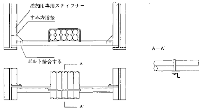
(図-5 添架用構造標準図)
