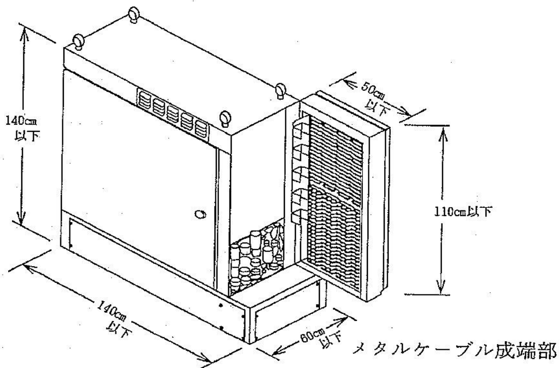
地上設置RT（1型）の外観図
