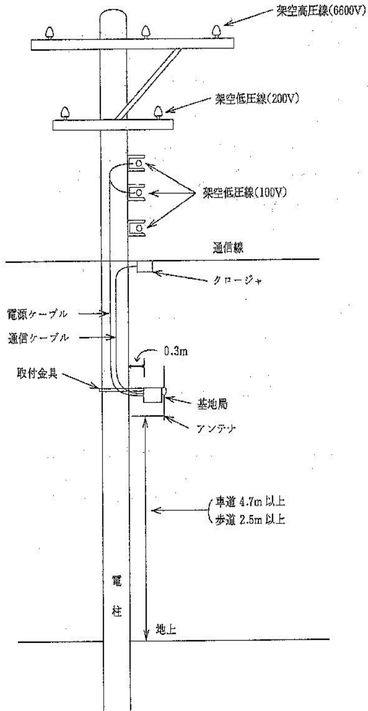
基地局取付図（標準） （100mW中間部） 通常設置の場合（アンテナが上下のもの）
