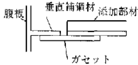
(図-4 ガセットと垂直補剛材の連結)
