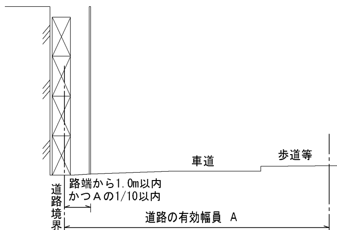
車道に設置する場合
