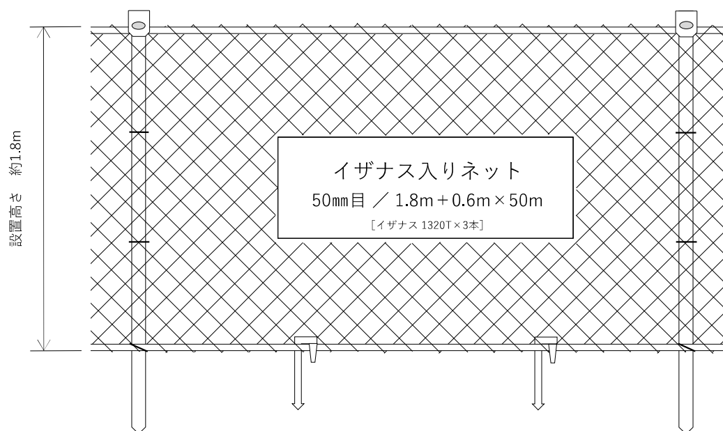
正面図
