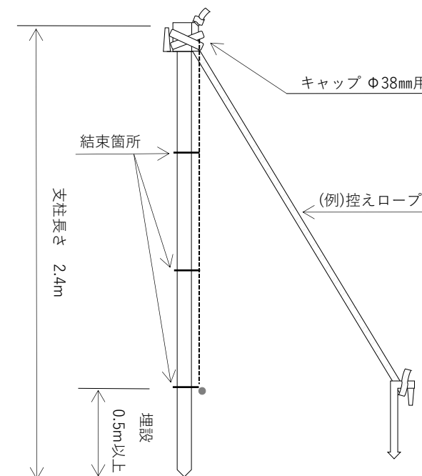
補強部 (例)
