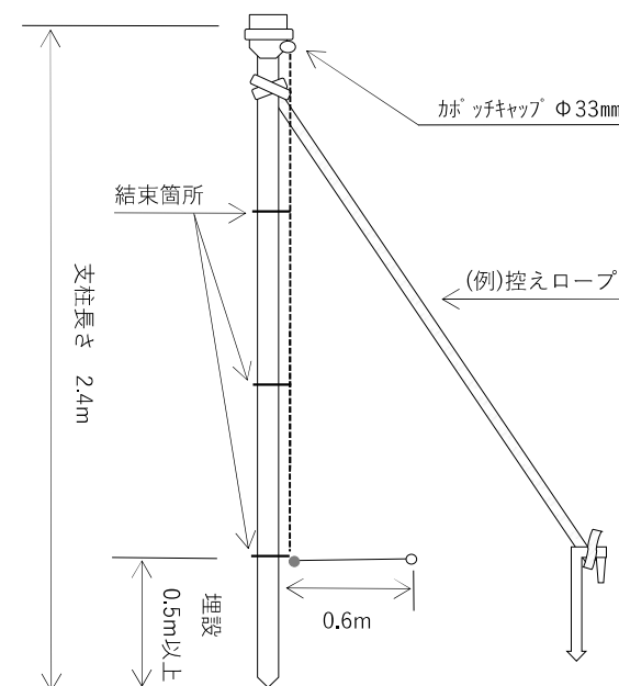
補強部 (例)
