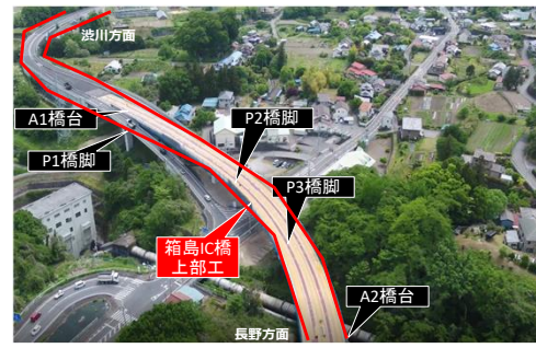
箱島IC橋(渋川方面) 施工状況 (R8.05撮影)
