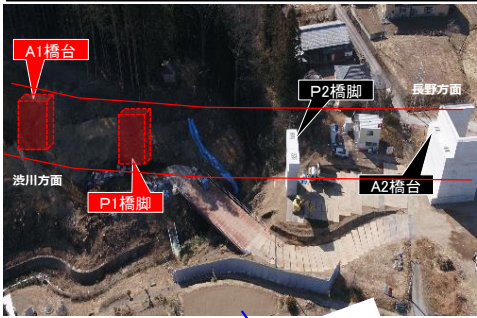
西沢橋 施工状況 (R8.05撮影)
