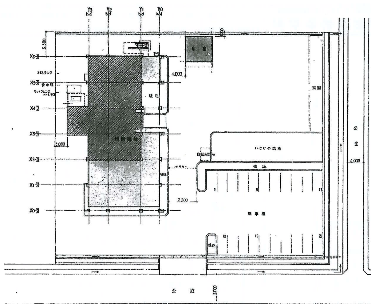
配置図 1:300
