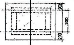
設備配管立上り口詳細図 1:30
