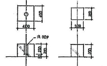
基礎A(4x4M) 基礎B(1x1M) クーリングタワー基礎詳細図 1:30
