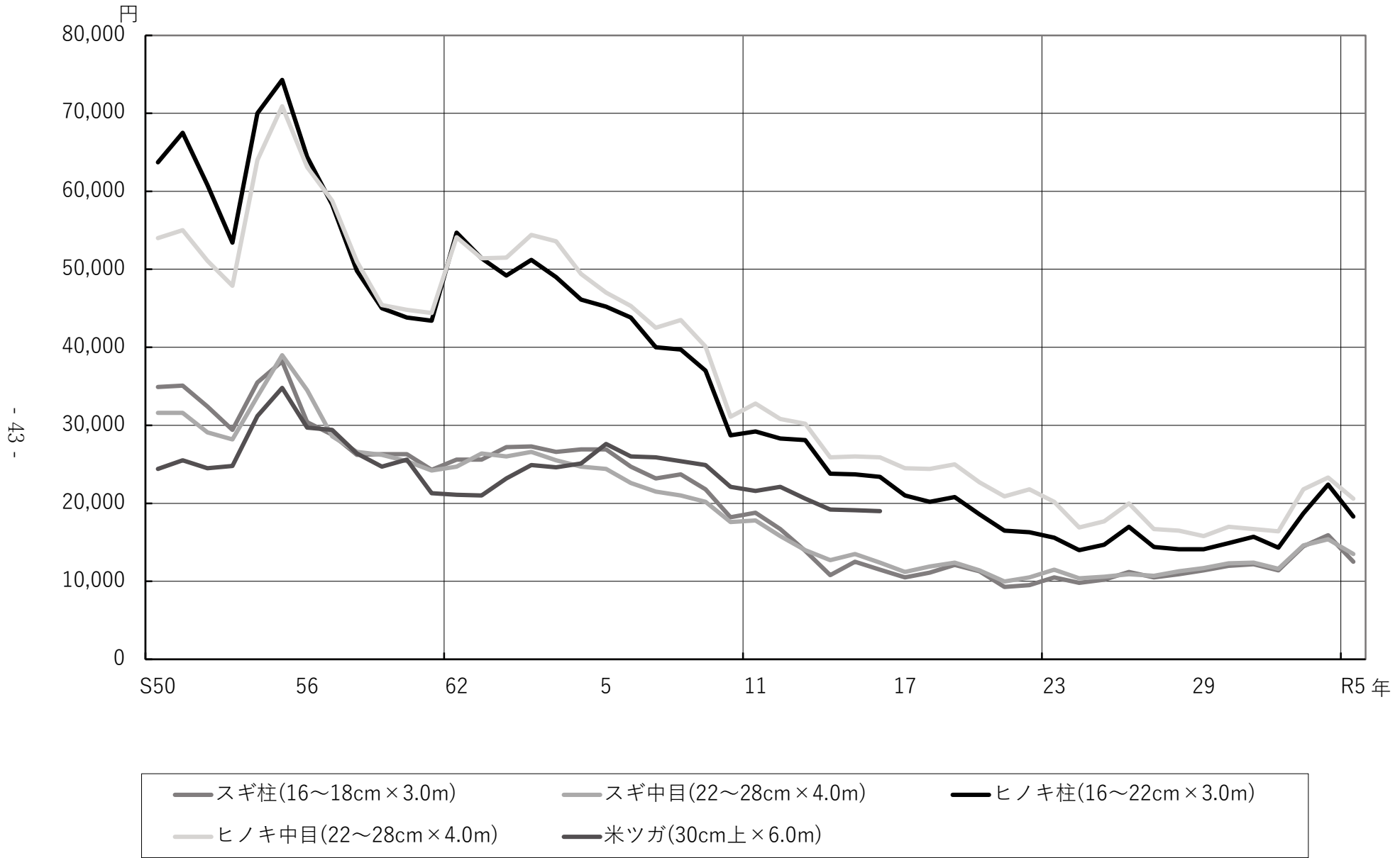
(2) 昭和50年からの推移 主要素材丸太 (年平均価格)
