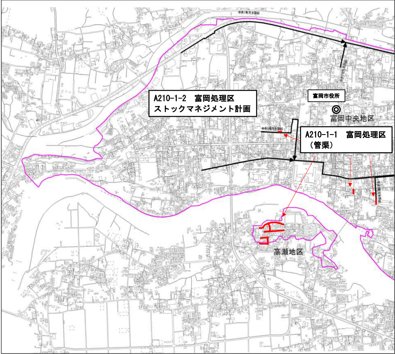
富岡市（県央処理区）計画図（1/2）
