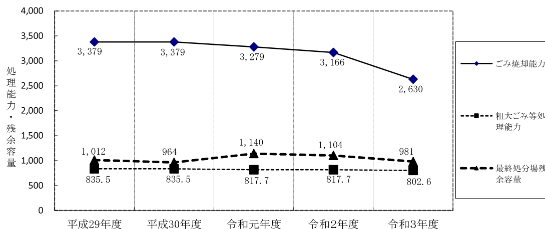
[図-1-11 ごみ処理施設整備の推移]
