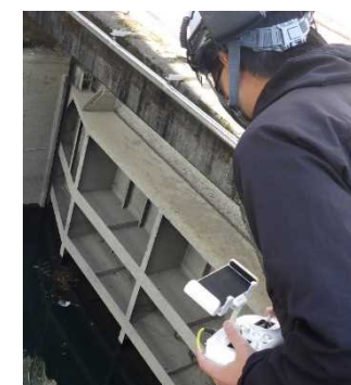
〔水中ドローンによる点検 (試行)〕
