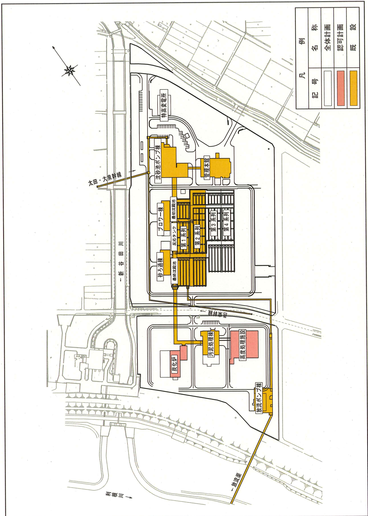
(3) 西邑楽水質浄化センター全体配置図
