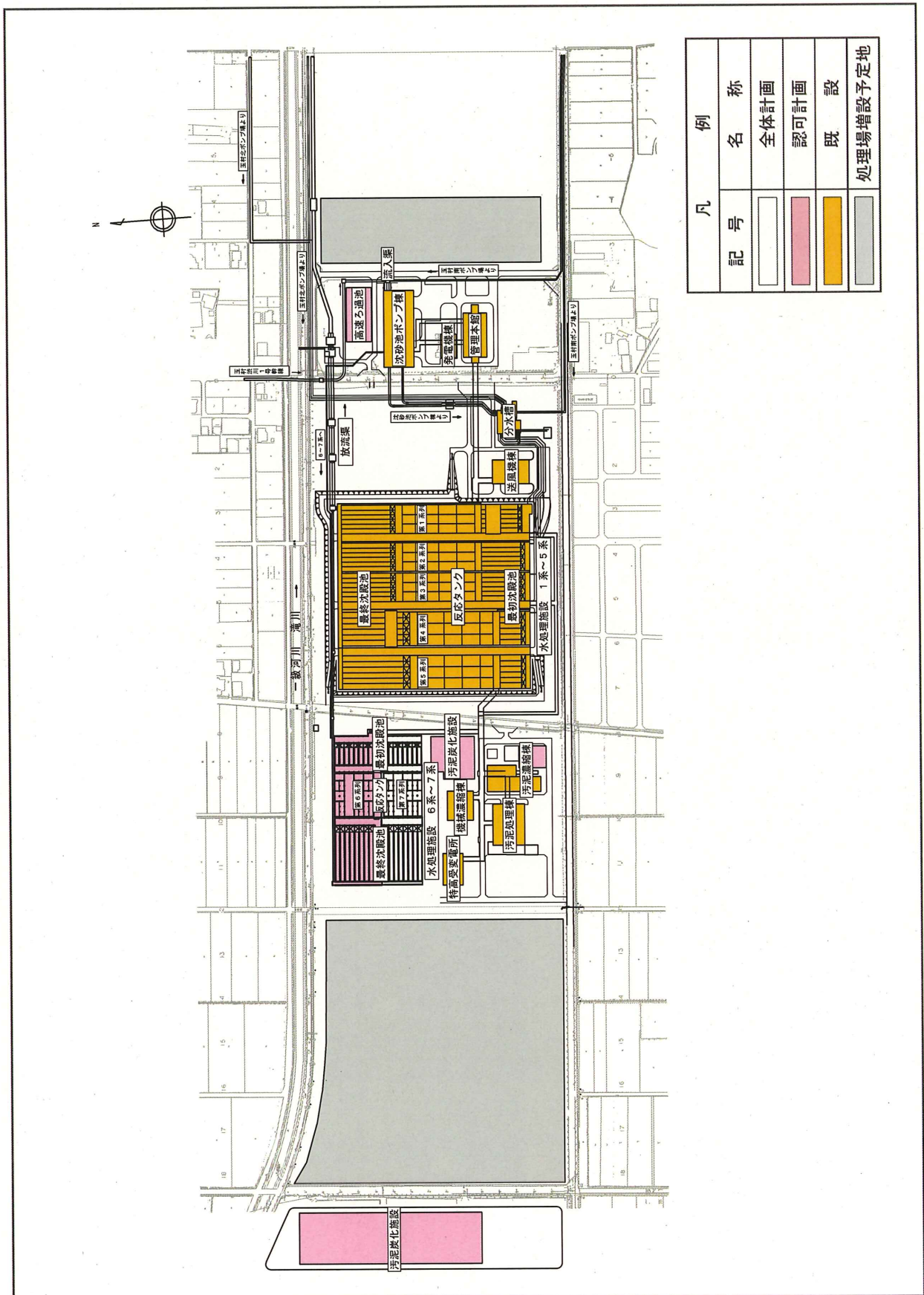
(3) 県央水質浄化センター全体配置図
