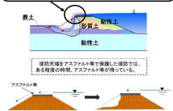
堤防天端舗装
