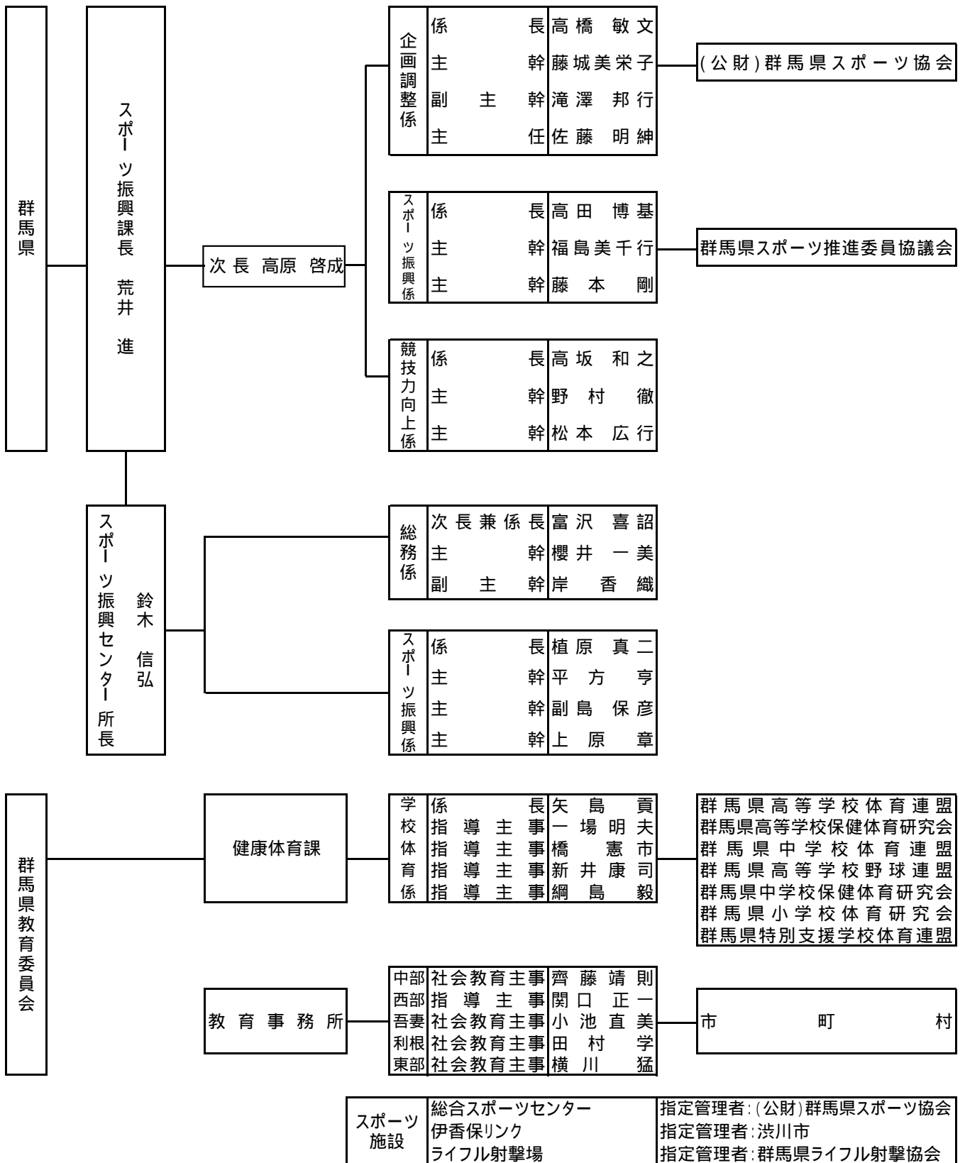
行政組織図
